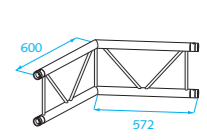
H40L-004U 120°
