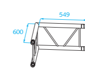
H40L-003U 90°
