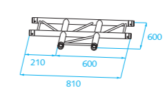
H40L-017F
