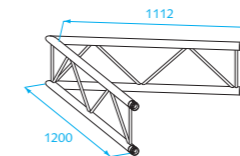
H40L-002U 60°
