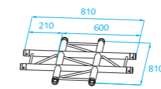
H40L-016F
