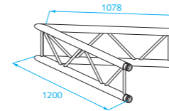
H40L-001U 45°
