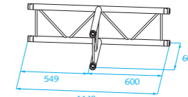
H40L-017U
